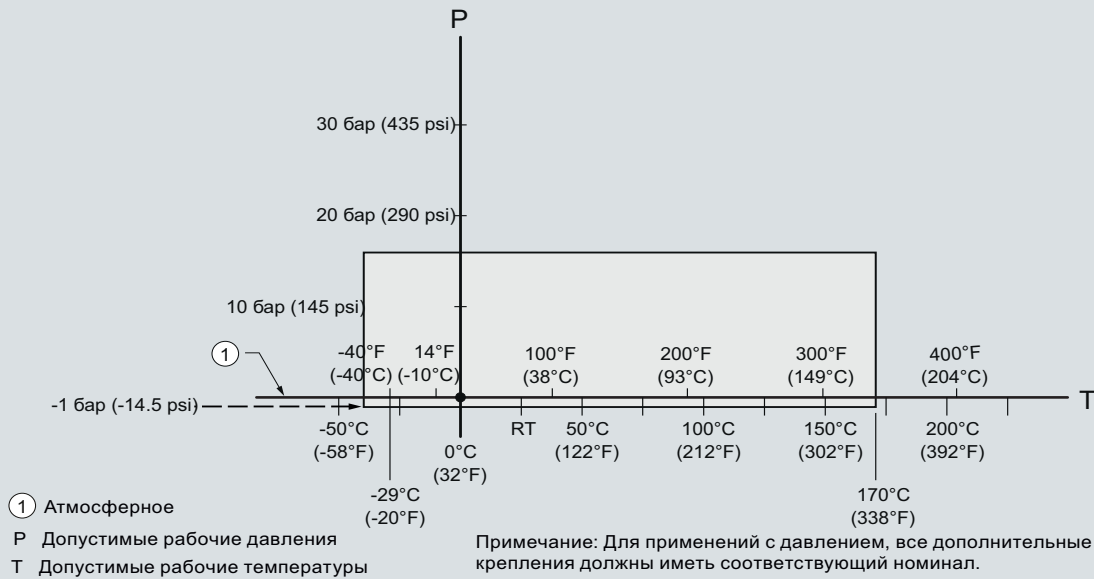
SITRANS LR250 с инкапсулированной гигиенической антенной, расчетные кривые давление процесса/температура
