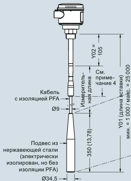
Модификация с кабелем, с изоляцией 3) Резьбовое соединение (7ML5673)
