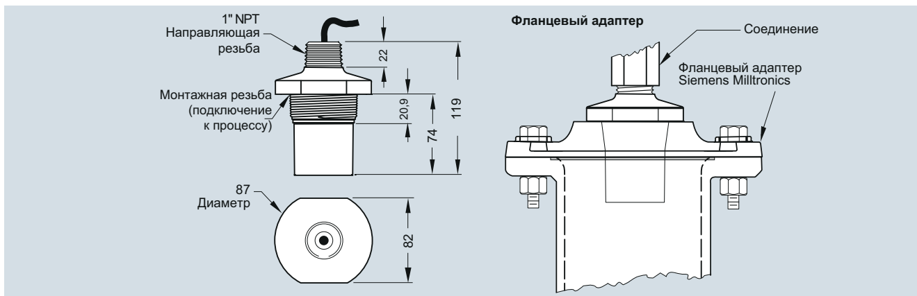
Ультразвуковой преобразователь ST-H, размеры в мм
