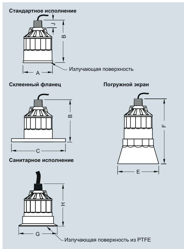
Ультразвуковой преобразователь XPS, размеры в мм
