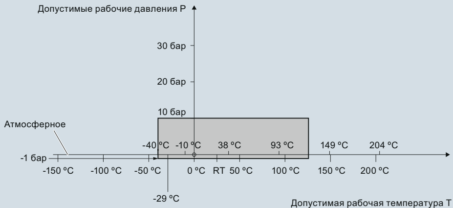
Pointek CLS200, кривые ухудшения параметров в зависимости от рабочего давления/температуры (7ML5632 и 7ML5642)
